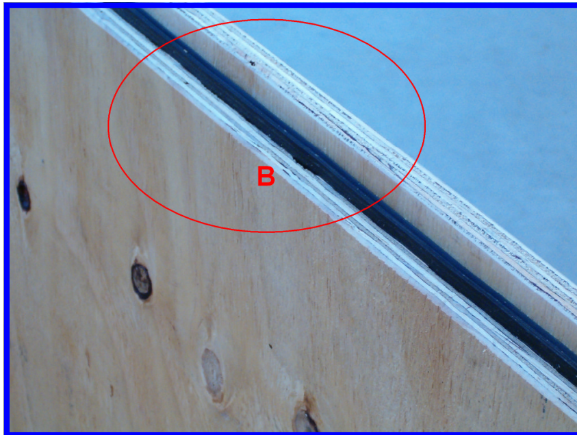
Bovenzijde rand archiefkist detail B toont de ingewerkte rubberen dichting .
